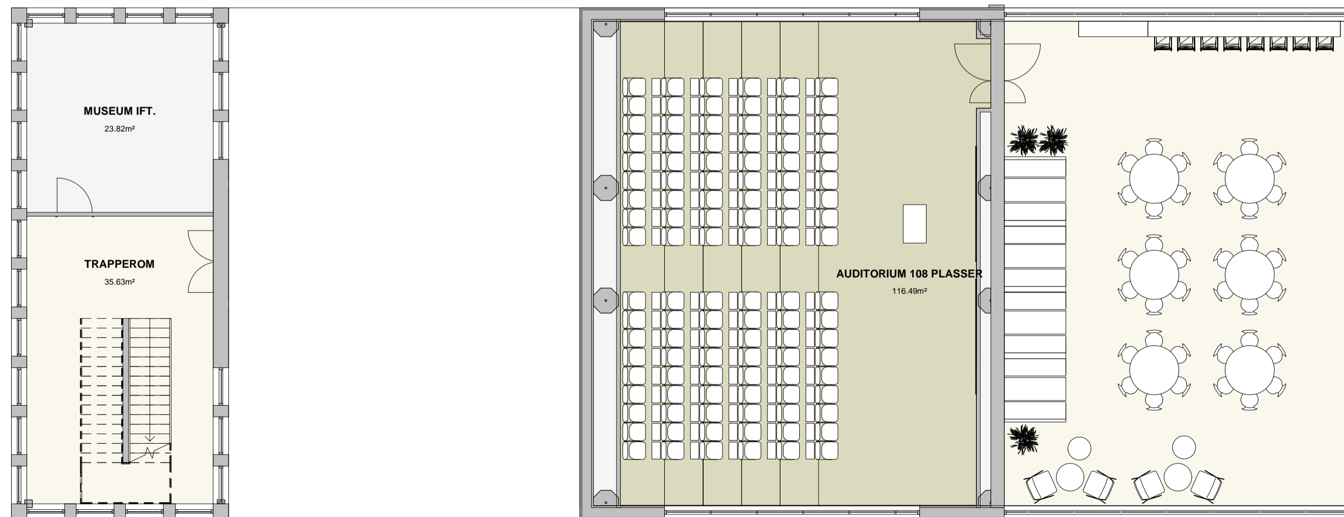
Plan 01 Endringsforslag 1 : 100
