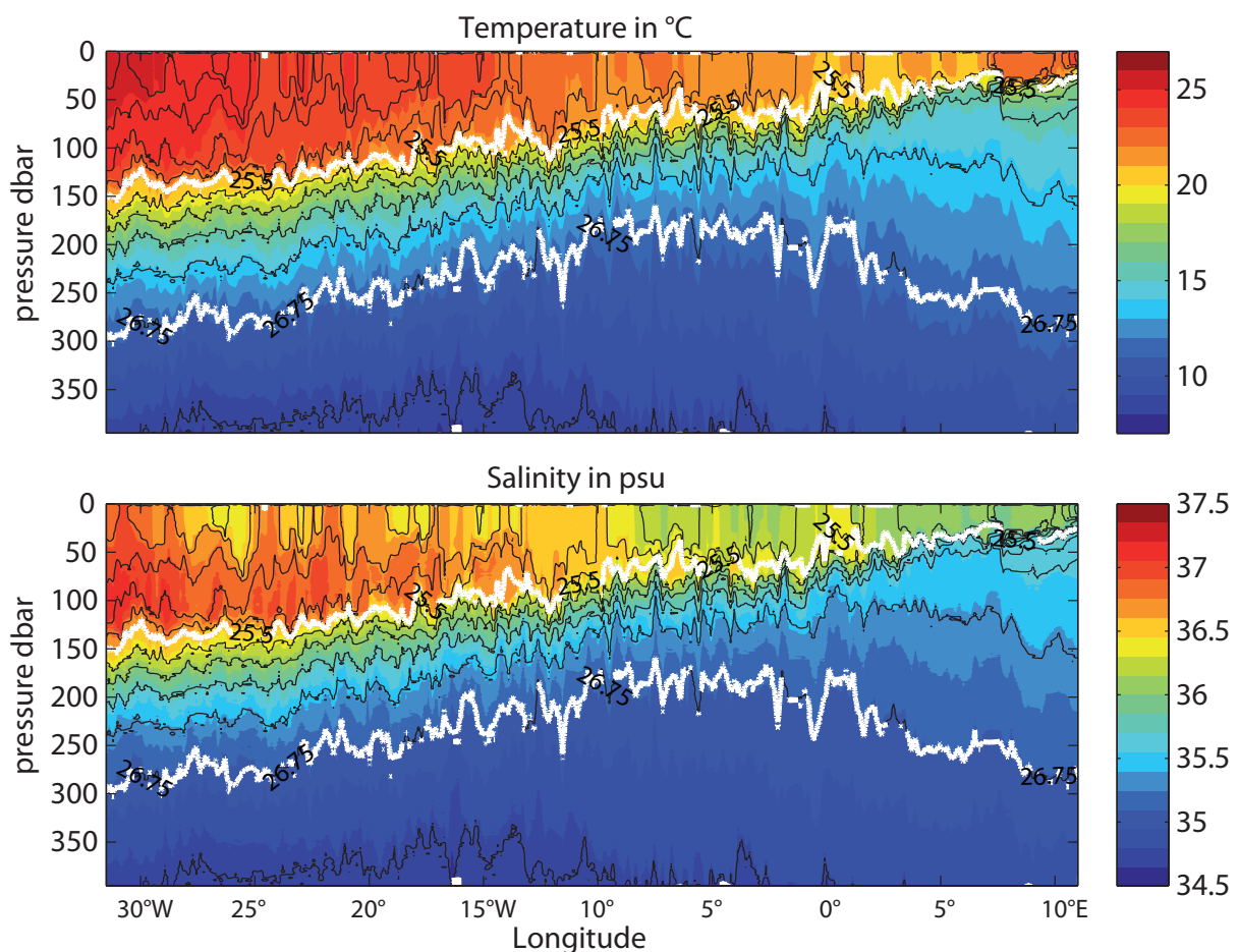
Abb. 1: Temperatur und Salzgehalt gemessen mit der Unterwegs-CTD entlang von \sim 11^{\circ}\text{S} von Brasilien bis Angola. Weiße und schwarze Linien sind Konturlinien der potentiellen Dichte (Abbildung: Sören Thomsen).
